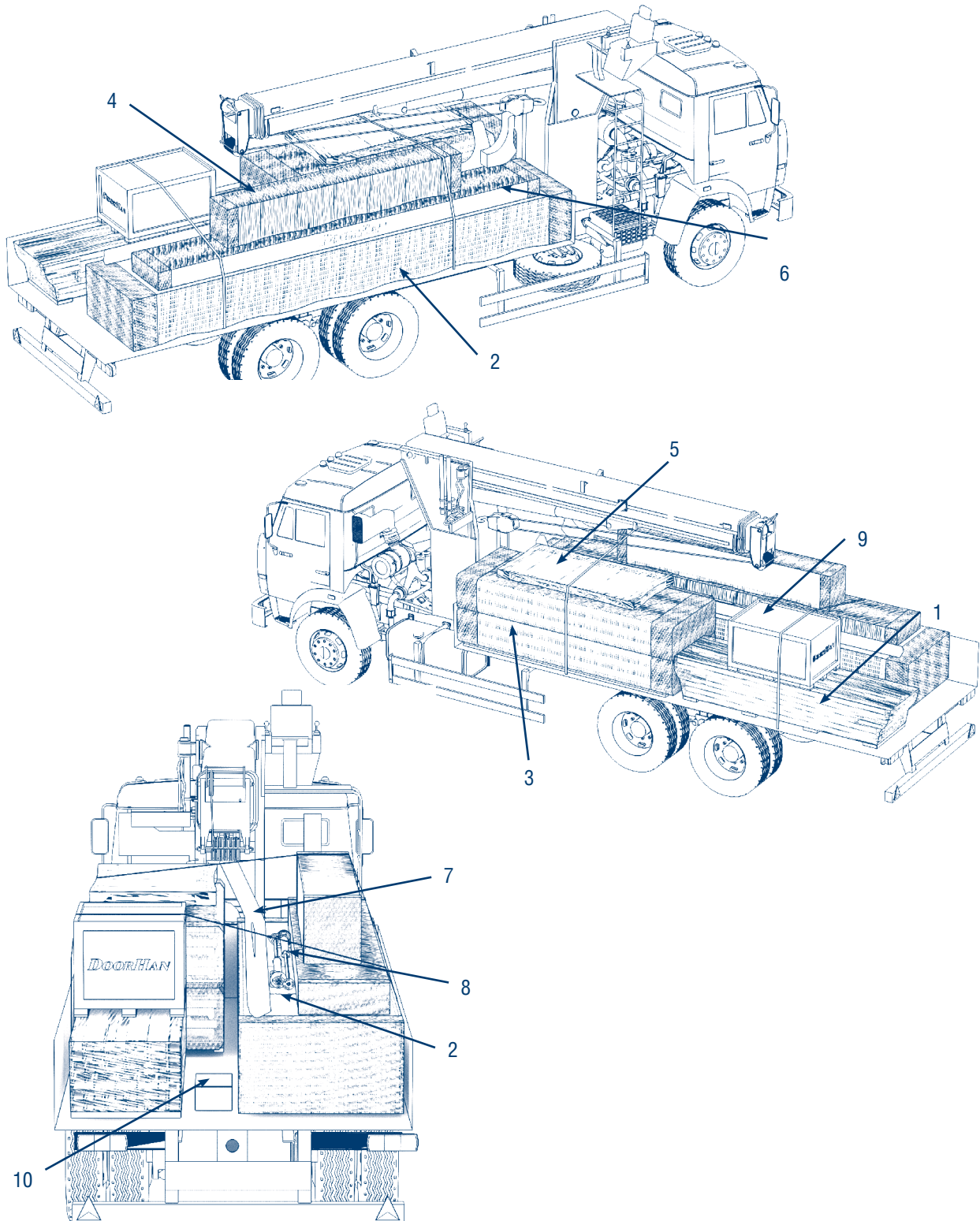
Рис. 6.2. Транспортировка комплектующих автотранспортом
