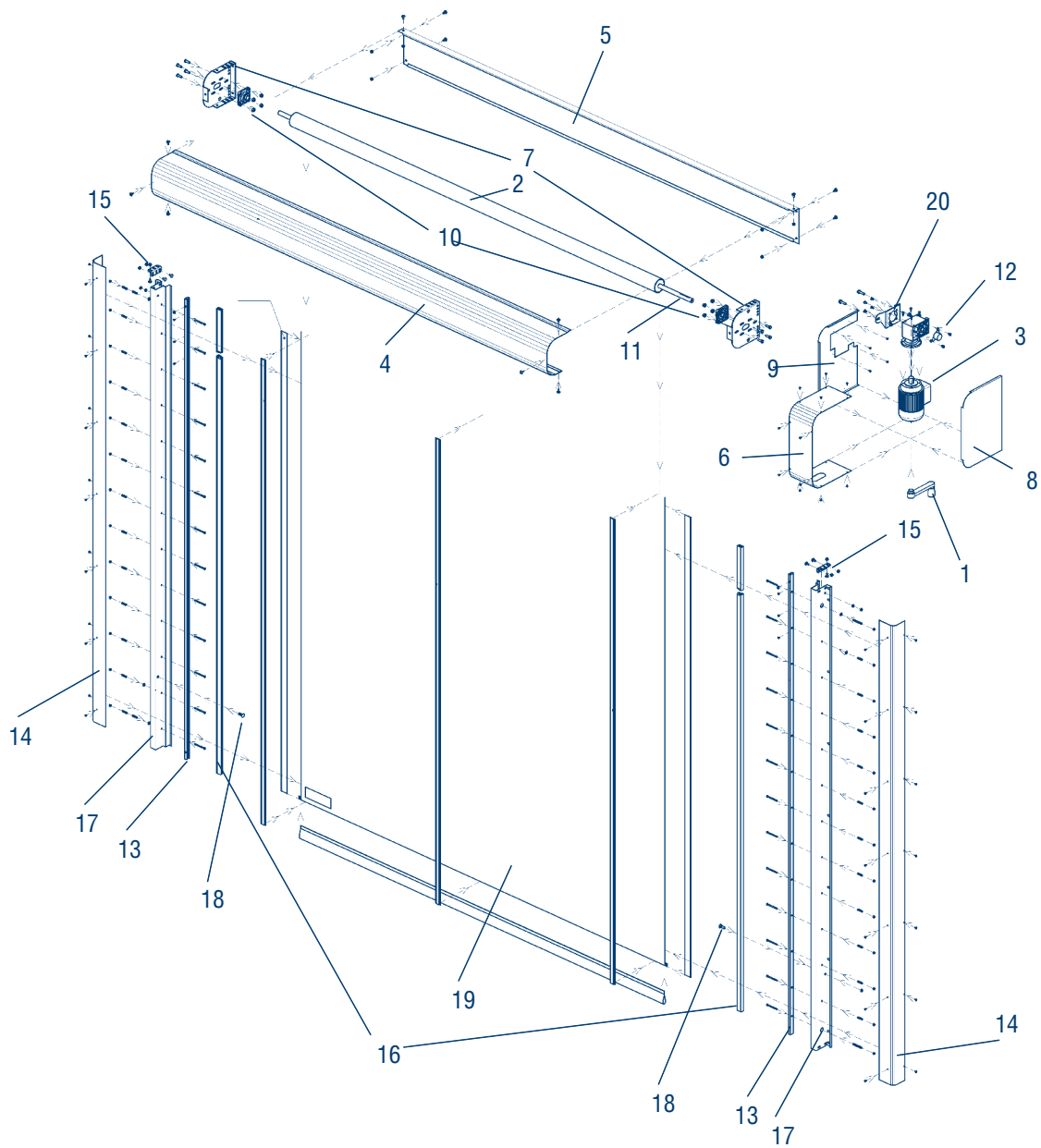
Рис. 1. Разнесенный вид
