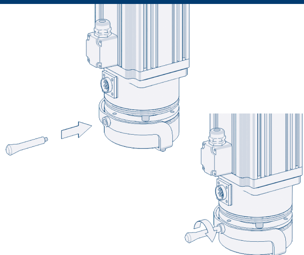
Рис. 3. Порядок установки рычага расцепителя тормоза
