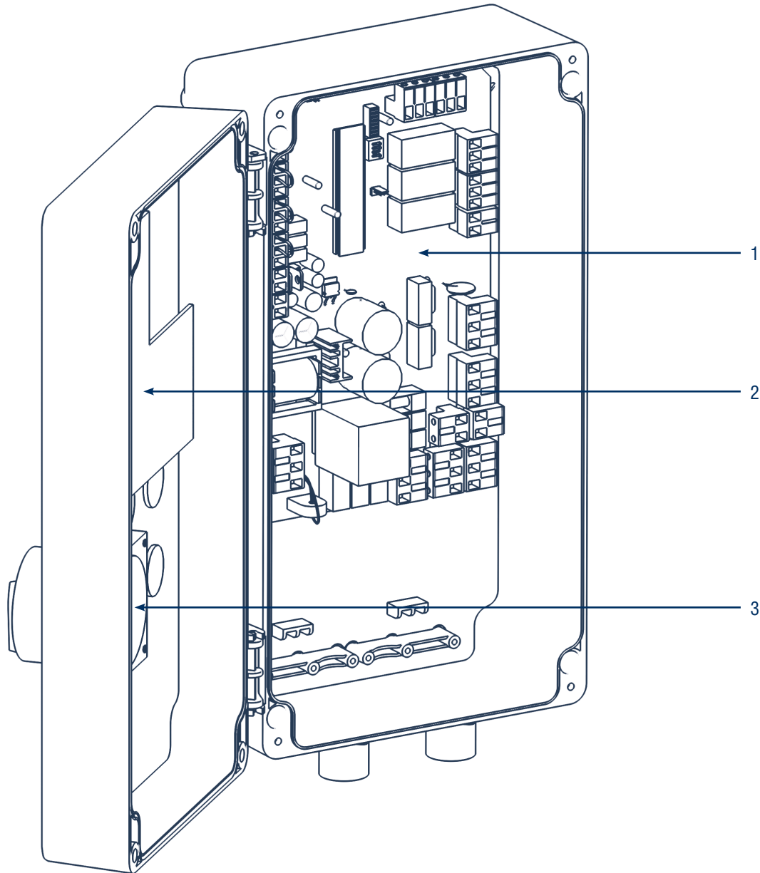
Рис. 1. Конструкция блока управления
